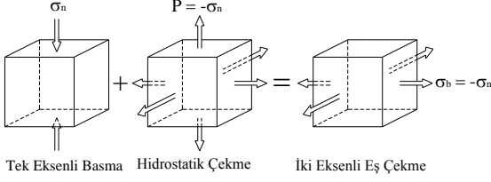
Şekil 33: Kauçuk türü malzemeler için iki eksenli eř çekme deformasyonunun elde edilmesi.
