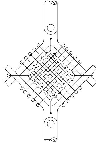
Şekil 35: Blatz ve Ko tarafından yapılan iki eksenli eř çekme deney düzeneęi.
