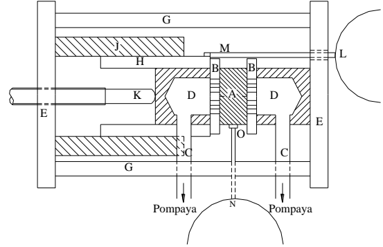
Şekil 54: Forster tarafından kurulan basit basma deney düzeni.
