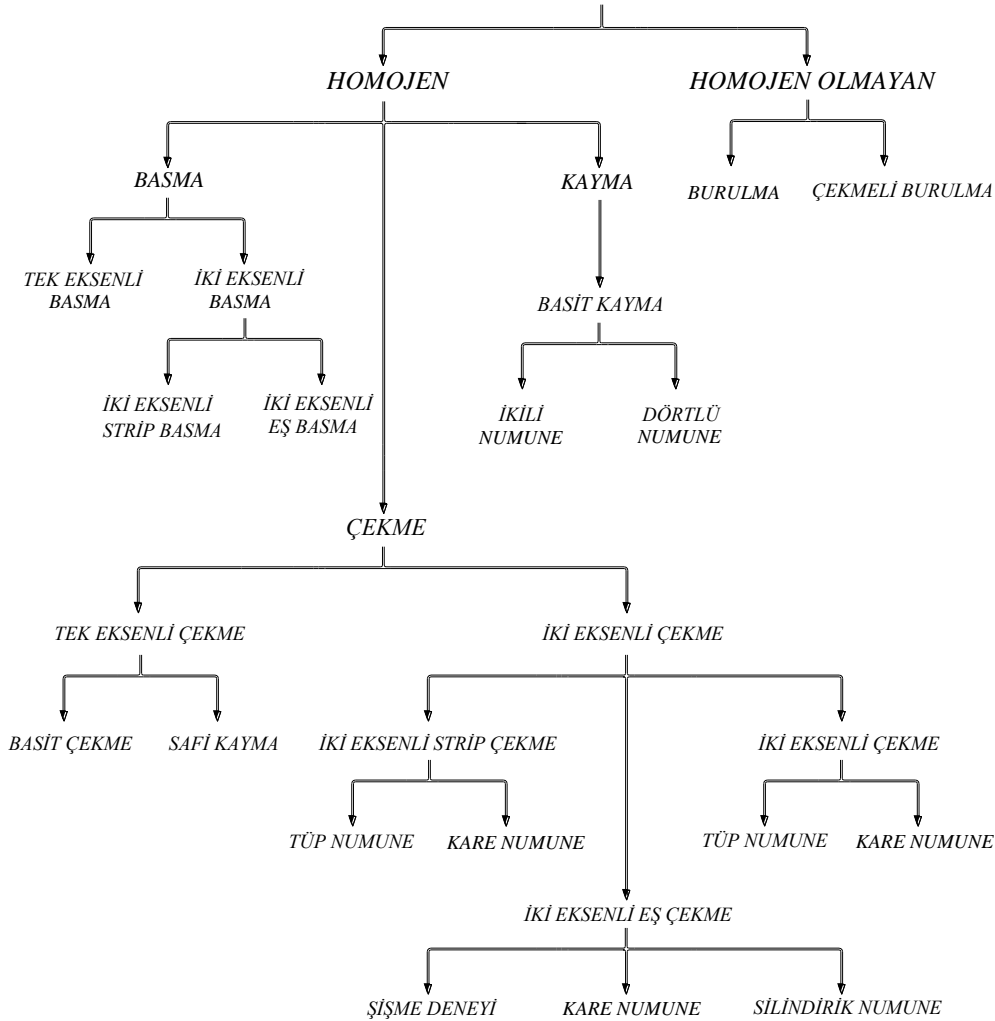
Şekil 1: Kauçuk mekanikinde yapılan deneyler [2].
