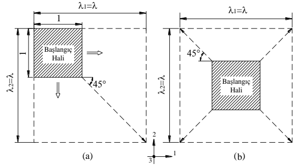
Şekil 34: Kare formdaki numunenin iki farklı durumda iki eksenli eř çekme deformasyon hali.
