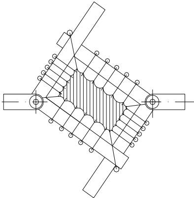
Şekil 17: Becker tarafından yapılan iki eksenli çekme deney düzeneği.
