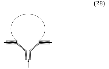
Şekil 41: Dairesel kauçuk membranın şişirilmesi deneyi.
