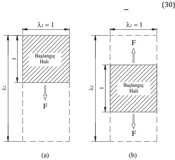
Şekil 47: Kare formdaki numunenin iki farklı durumda iki eksenli strip çekme deformasyonu.
