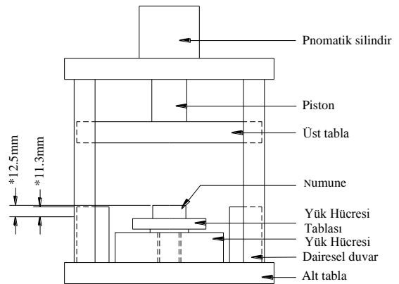
Şekil 55: Yeoh tarafından kurulan basit basma deney düzeni.
